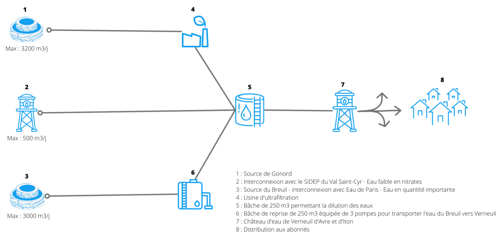
Distribution de l'eau potable sur la commune de Verneuil d'Avre et d'Iton Schéma de fonctionnement
